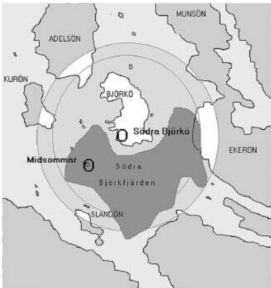
Meteoritkraterns utbredning i Södra Björkljärden. De dubbla ringarna indikerar osäkerheten för kraterns utbredning.
